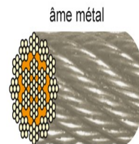
19 x 7 fils
