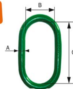
ANNEAU SIMPLE ref. 5058 Pour élingues-câble 1 et 2 brins
