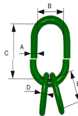
ANNEAU TRIPLE ref. 5059 Pour élingues-câble 3 et 4 brins
