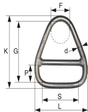
ANNEAU FEMELLE ref. 5072
