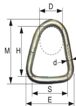
ANNEAU MÂLE ref. 5070
