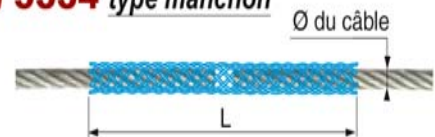
réf 5334 type manchon
