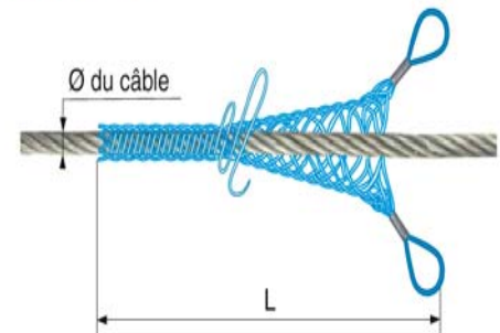
réf 5337 double-boucle à lacet
