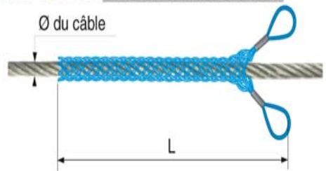
réf 5336 ouvert / double-boucle
